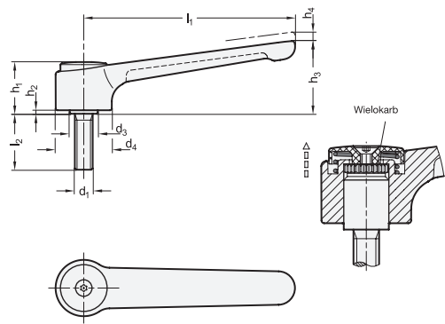
GN 126-Trzpień gwintowany
